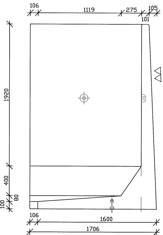
aanzicht B-B
