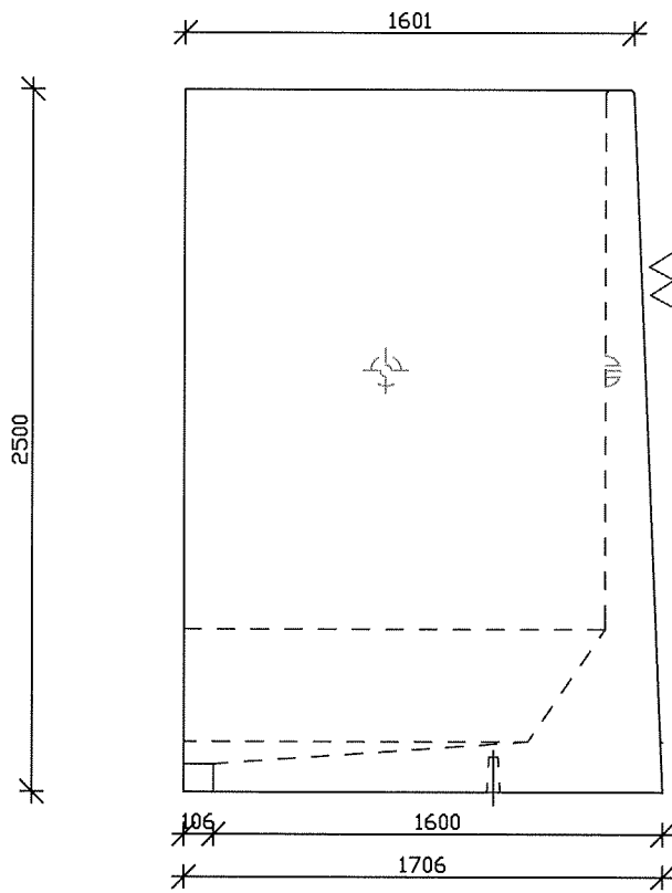
aanzicht A-A
