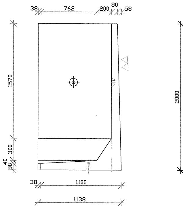
aanzicht B-B
