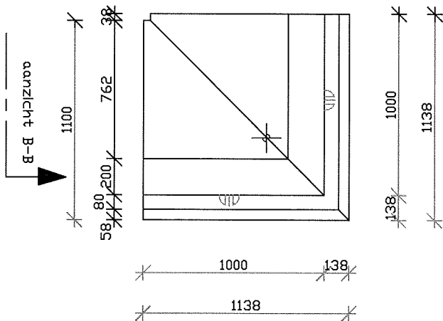
aanzicht A-A
