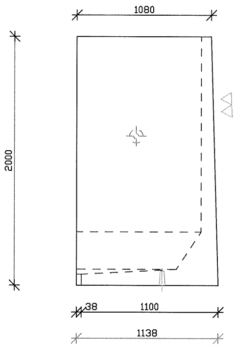
aanzicht A-A
